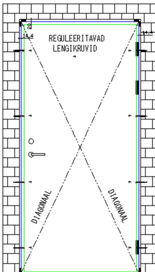
Joonis 1. Ukselengi fikseerimine ehitusavasse.
